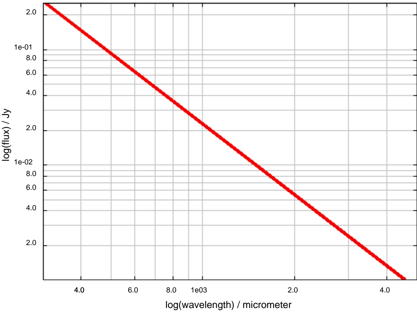
Alpha Cetus (Decin Flux Model)
